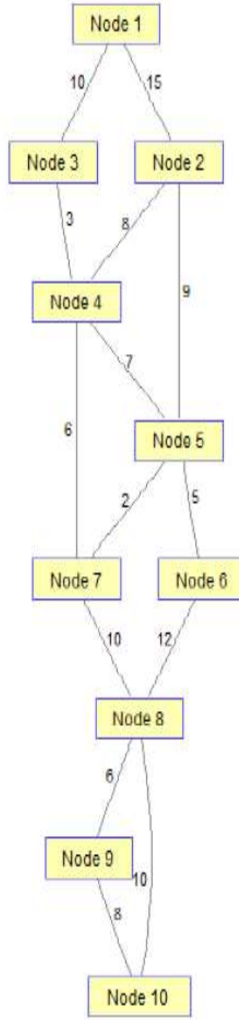
Fig. 3.0 OSPF ALONE
