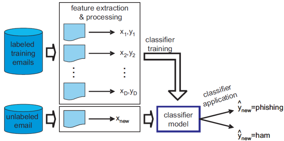
Fig 4.0: Machine Learning Approach (Bergholz et al, 2008)
